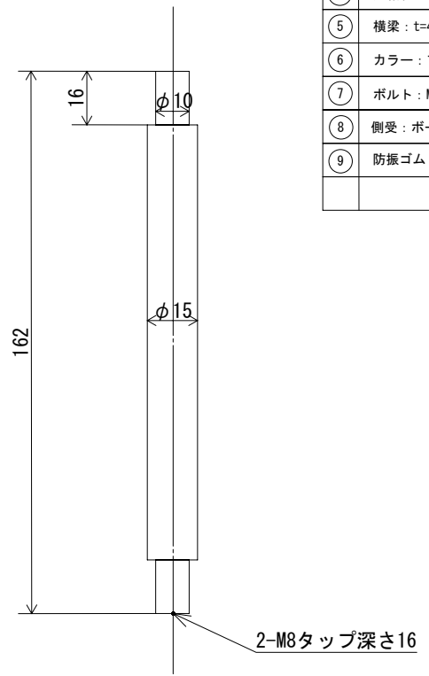
④ 連結軸部品図
