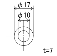
⑥ カラー部品図
